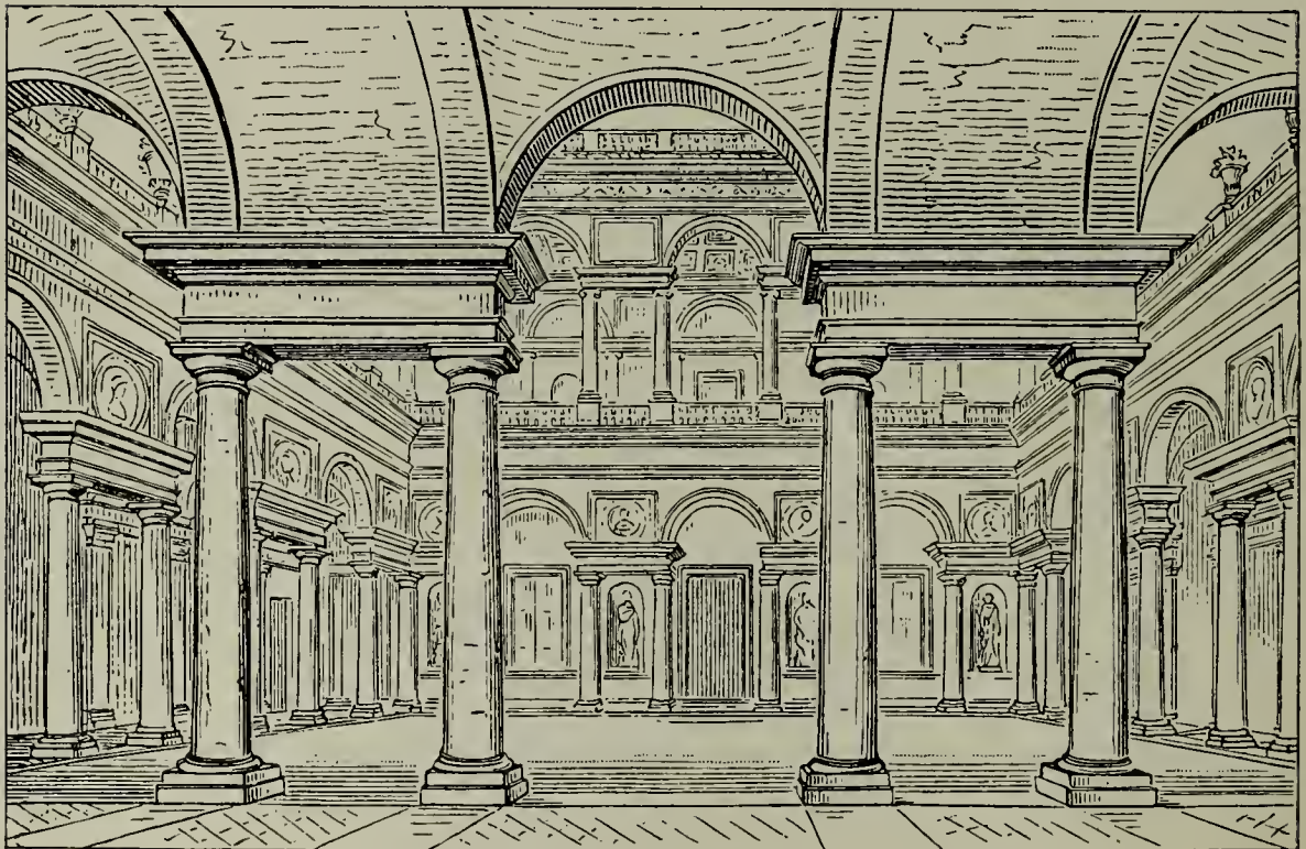
Abb. 238. Ehemaliger Hof von Pal. Sauli zu Genua.
